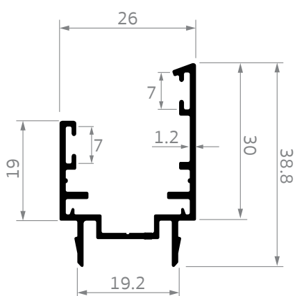
SS-X213 เสริมเสากันแฉกเข้ามุม (ตัวเมีย) สมาร์ต เอ็กซ์
