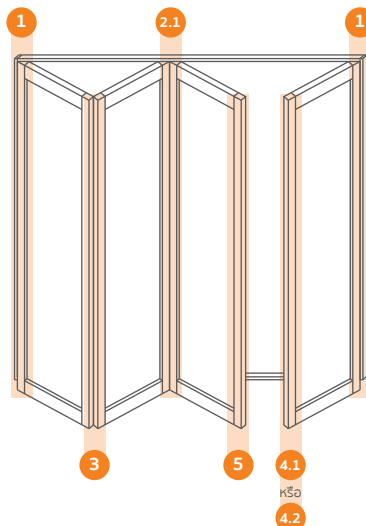
บานเฟี้ยมคี่ (ปิดชนกลาง)
