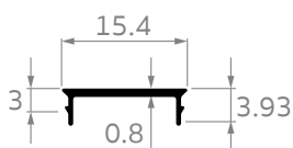
SC-X105 ฝาปิดร่อง C-18 สมาร์ท เอ็กซ์
