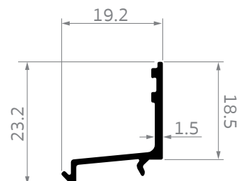
SF-X106 คิ้วช่องแสง, บานเปิด ร่อง 32.5 มม. สมาร์ท เอ็กซ์
