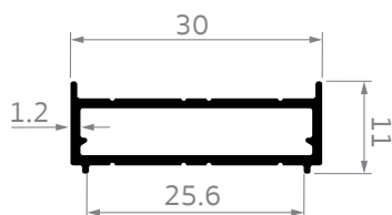
iO-0210 เฟรมระแนง 30x11 ไอคอนิก
