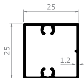
iO-0209 กล่องระแนง 25x25 มีรูสกรู ไอคอนิก
