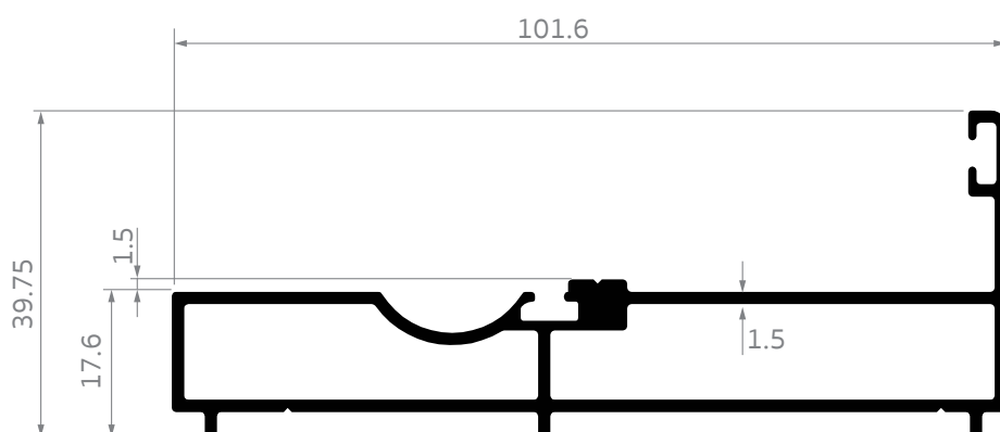
SB-0105 เฟรมข้าง บานเฟี้ยม สมาร์ท เอ็กซ์
