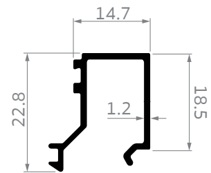
SF-X111 คิ้วช่องแสง, บานเปิด ร่อง 20 มม. สมาร์ท เอ็กซ์
