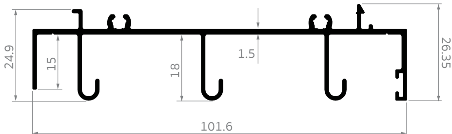
SS-X104 ทูบเฟรม 3 รางบานเลื่อน ต่อช่องแสง สมาร์ท เอ็กซ์
