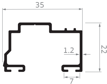
iO-0206 เสริมขวางล่างประตู บานเปิด ไอคอนิก
