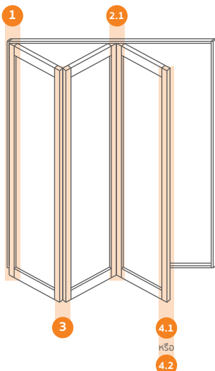
บานเฟี้ยมคี่ (เปิดทางเดียว)
