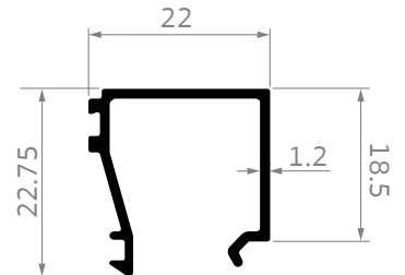
SF-X108 คิ้วช่องแสง, บานเปิด ร่อง 12.7 มม. สมาร์ท เอ็กซ์
