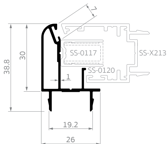
SS-X214 เสริมเสากันแฉกเข้ามุม (ตัวผู้) สมาร์ต เอ็กซ์
