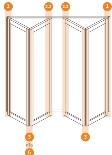
บานเฟี้ยมคู่ (ปิดชนกลาง)
