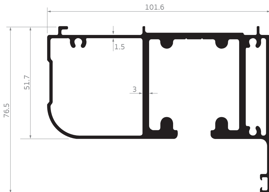
SB-0101 เฟรมบน บานเฟี้ยม สมาร์ท เอ็กซ์
