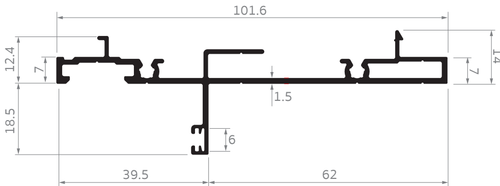
iC-0110 ตบเฟรมบานกระทุ้ง ซิกูฟนอก ไอคอนิค
