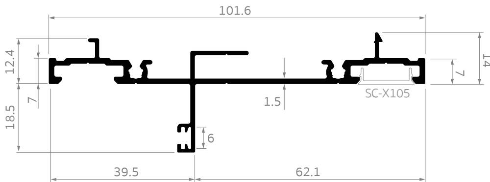
SC-X104 ตบเฟรมบานกระทุ้ง สมาร์ท เอ็กซ์
