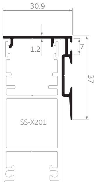
SS-0139 ตบเกี่ยวทางเดียว สมาร์ต เอ็กซ์
