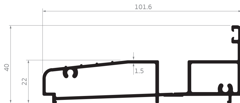
SB-0103 เฟรมล่าง บานเฟี้ยม สมาร์ท เอ็กซ์
