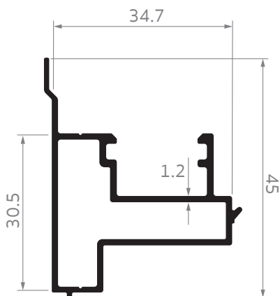
SC-0212 เสริมเสาบานเปิดคู่ สมาร์ท เอ็กซ์
