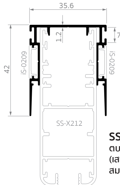
iS-0209 ฝาปิดสกรูตบเกี่ยว โอคอนิค
